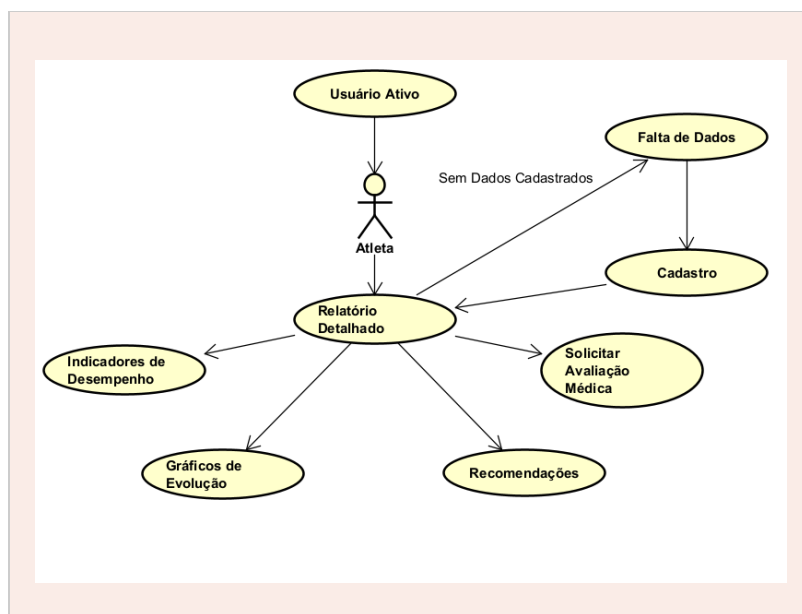
Figura 4 - Diagrama de Casos de Uso - Atleta / Jogador.
