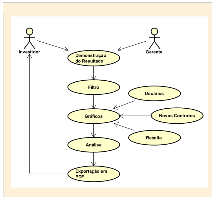
Figura 7 - Diagrama de Casos de Uso - Investidor / Painel Executivo.
