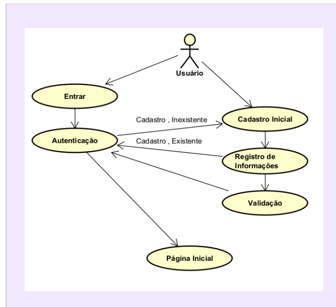
Figura 1 - Diagrama de Casos de Uso - Acesso ao Sistema.
