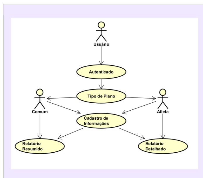
Figura 2 - Diagrama de Casos de Uso – Usuário Comum / Atleta.
