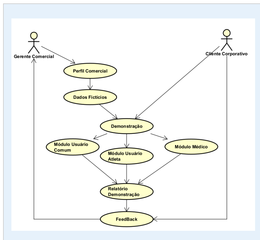
Figura 5 - Diagrama de Casos de Uso - Gerente Comercial / Vendas.
